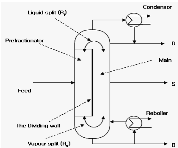
그림 5. 분리벽형 증류탑(DWC) 구성도. Fig. 5. Structure of dividing wall column.
