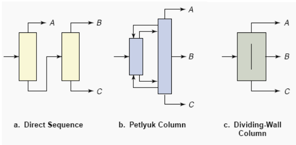
그림 8. 3성분 분리를 위한 증류구조. Fig. 8. Distillation process for ternary mixture separation.
