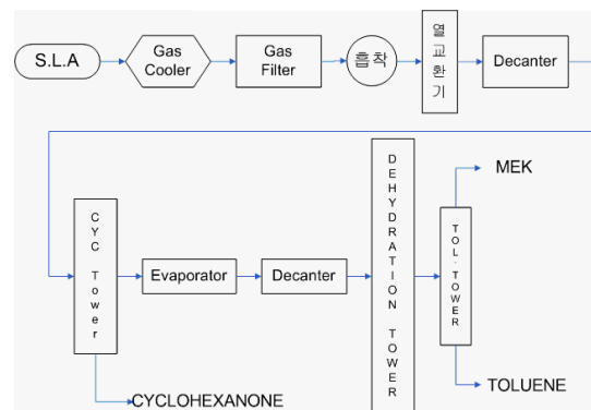
그림 1. 기존의 용매회수 공정 블록선도.
